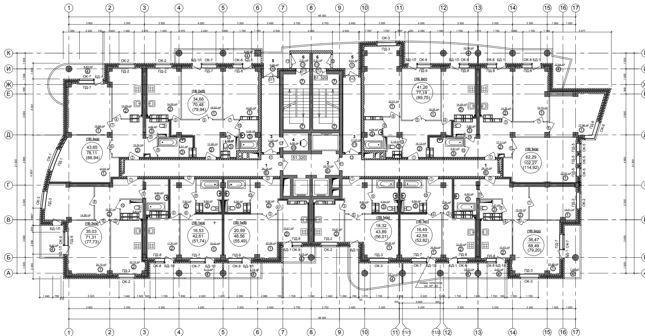
Экспликация помещений общественного пользования жилой части дома на 18 этаже
